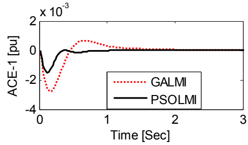
(d) ACE in area-1
