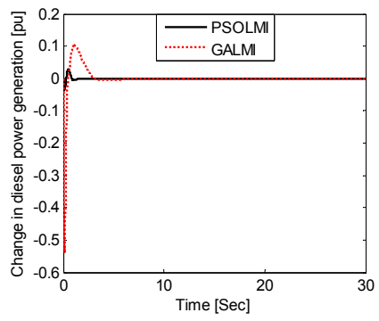
(d) Change in diesel power generation
